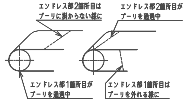
プリー部でのエンドレス部の位置関係イメージ
